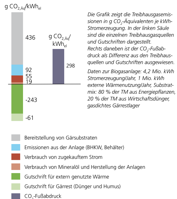
Abb. 23: Ergebnisdarstellung der Klimagasbilanz für eine Biogasanlage mit 500 kW el (Quelle: LWK Niedersachsen)
