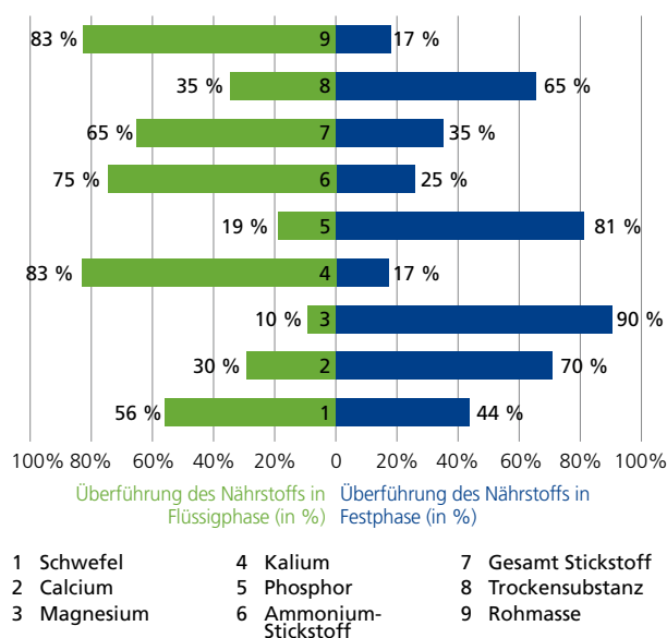
Abb. 22: Nährstoffverteilung für die Separation von Mastschweinegülle mit der Zentrifuge der Raiffeisen-Warengesellschaft Emsland-Süd eG
