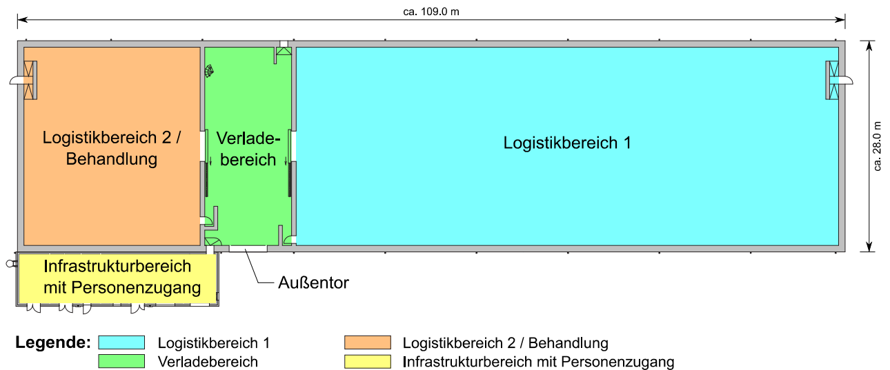
Abbildung 3-2: Funktionsbereiche des TLE
