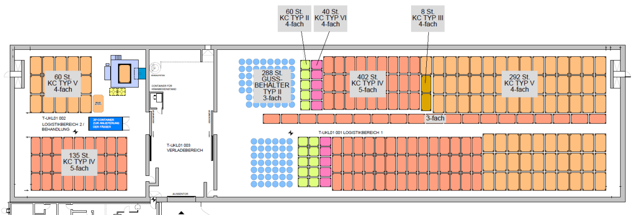
Abbildung 4-3: Beispielbelegung des TLE mit Gebinden und Mobiler Beladestation
