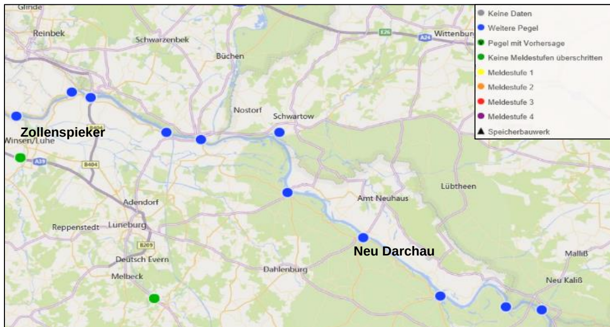
Abbildung 6: Auszug aus Pegelonline Niedersachsen (verändert nach NLWKN 2019b)
