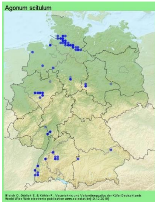
Abbildung 28: Verbreitung von Agonum scitulum (BLEICH et al. 2019)
