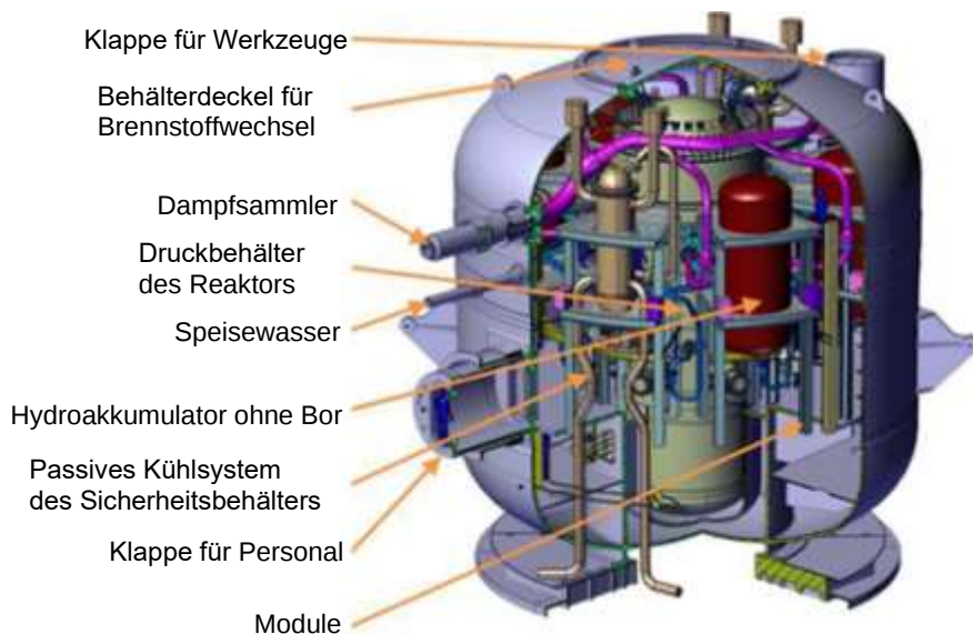
Abb. B.12: Querschnitt durch den NUWARD-Innensicherheitsbehälter
