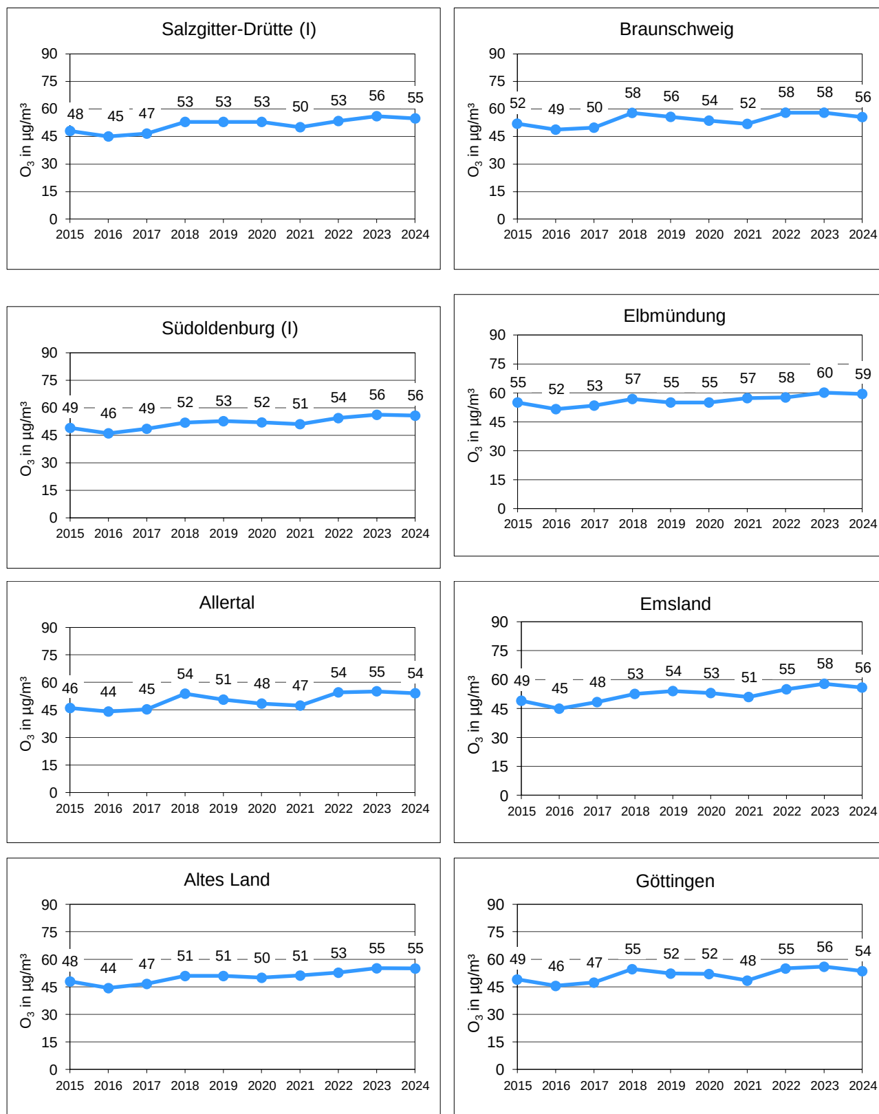
Diagramme C8: Jahresmittelwerte Ozon (O 3 ) – Industrienah und im städtischen, vorstädtischen und ländlichen Hintergrund
