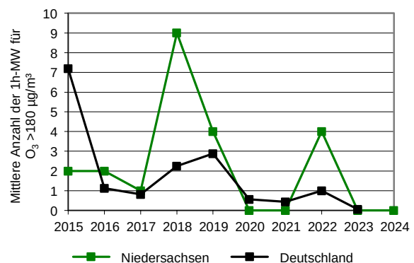
Abbildung E4: Mittlere Anzahl der O_3 -Stundenmittelwerte > 180 \mu g/m^3 pro Jahr im städt. Hintergrund
