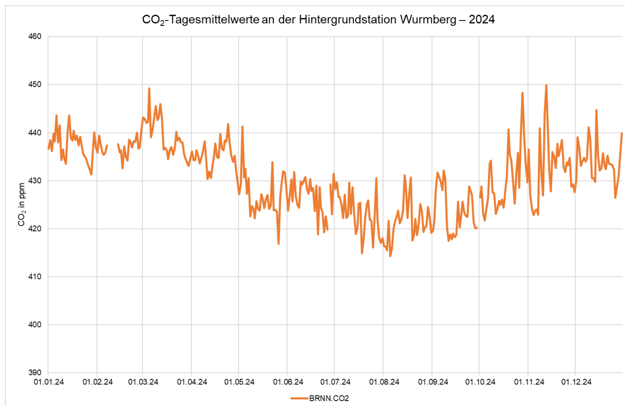
Abbildung I4: CO 2 -Tagesmittelwerte an der Hintergrundstation Wurmberg im Jahr 2024
