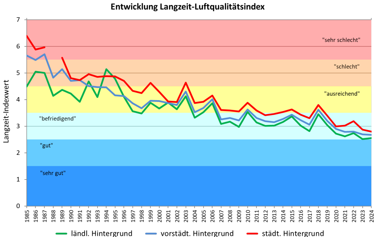
Abbildung D5: Langzeit-Luftqualitätsindexe (L-LQI) 1985 bis 2024
