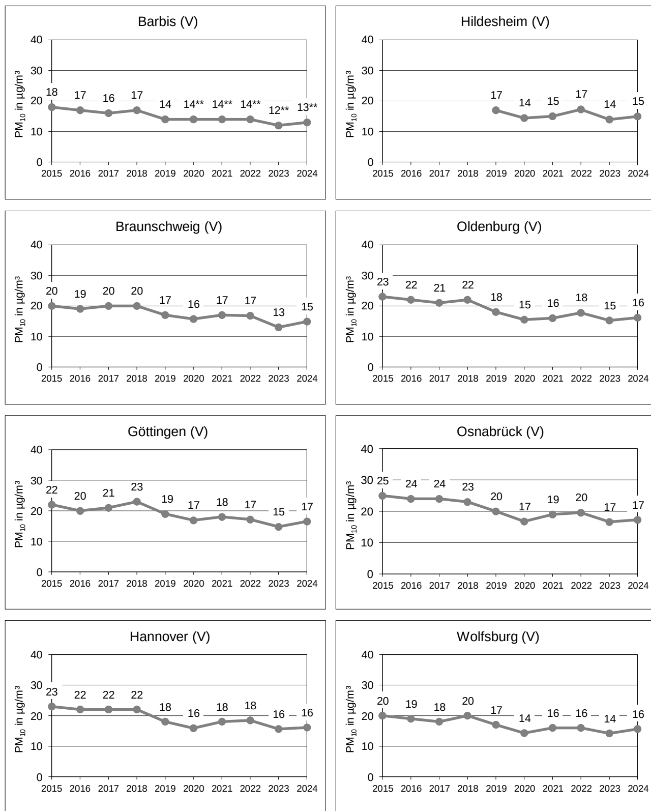
Diagramme C4: Jahresmittelwerte Partikel PM 10 – Verkehrsnah
