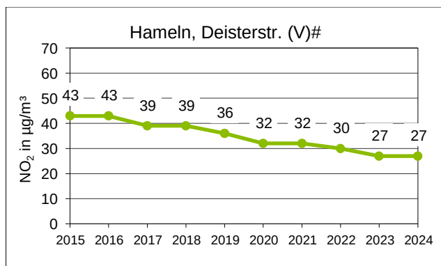
Diagramme C2: Jahresmittelwerte Stickstoffdioxid (NO 2 ) – Verkehrsnah
