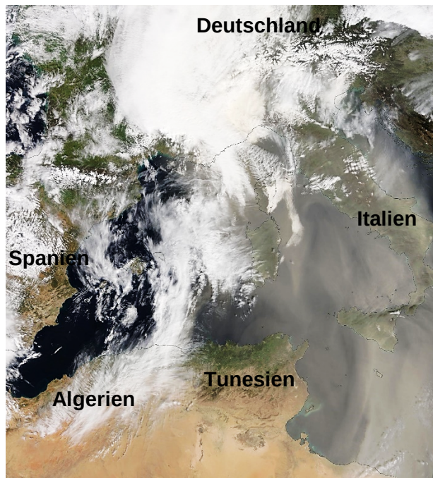
Abbildung 2.2: Satellitenbild am 30.03.2024. Am unteren Bildrand sind Teile Algeriens und Tunesiens zu sehen, am rechten Bildrand Italien, am linken Bildrand der Osten Spaniens. Deutschland ist unter den Wolken im oberen Bildbereich nicht zu erkennen. Deutlich sichtbar ist hingegen ein breites Band aus Saharastaub, welches sich östlich von Tunesien bis nach Italien erstreckt.
