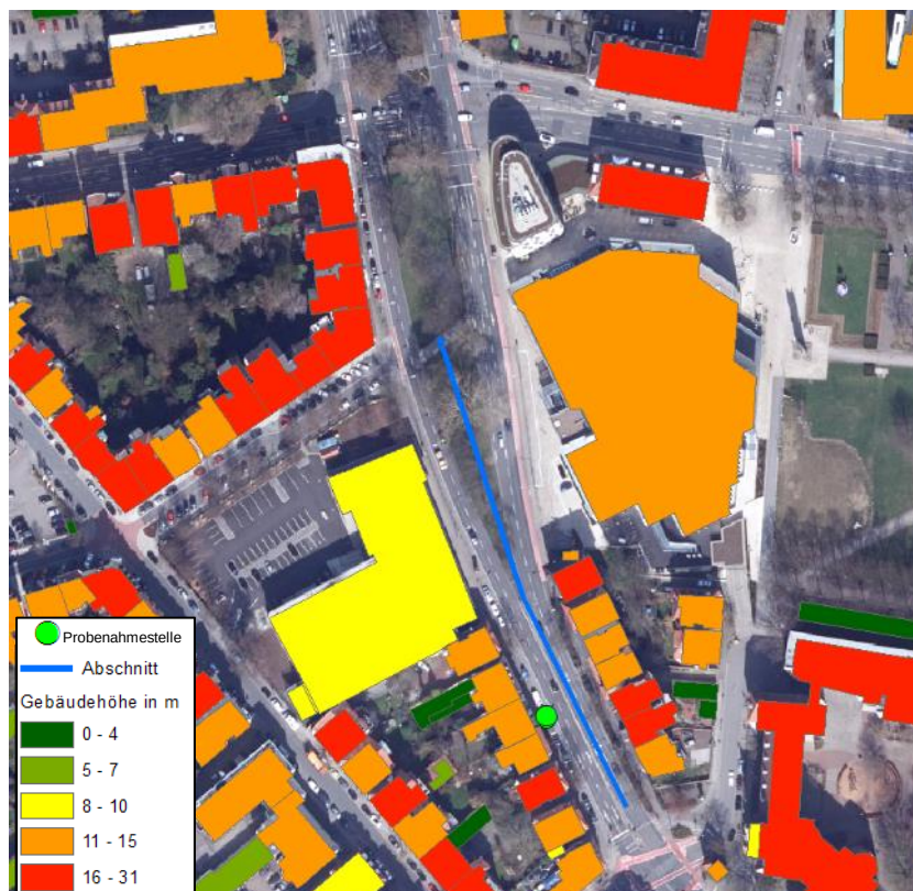
Abb. A.10: Lage des untersuchten Abschnitts am Schloßwall in Osnabrück mit Standort der Probenahmestelle (DENI067)
