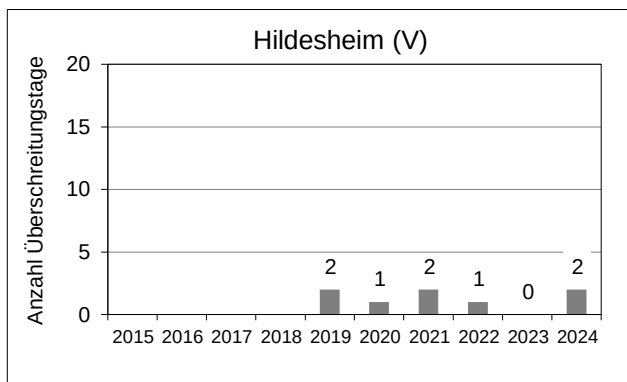
Diagramme C5: Anzahl Tage mit Tagesmittelwerten >50 \mu\text{g}/\text{m}^3 für Partikel \text{PM}_{10} – Verkehrsnahe
