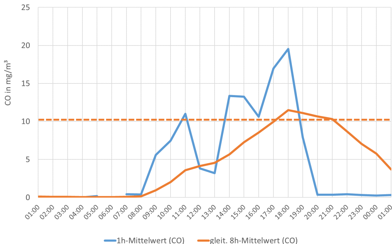
Abb. 1: 1h-Mittelwerte und gleitende 8h-Mittelwerte für CO am 28.05.2024 an der Messstation DENI067
